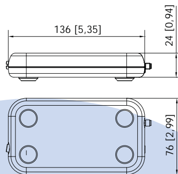
PErL (mm [inches])
